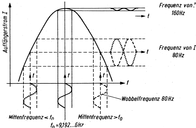
Bild 5. Ausschnitt aus der Resonanzkurve des CS-Resonators; Prinzip der Ableitung des Korrektursignals
