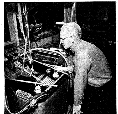
Bild 6. Der holografische Film, wird, um einen Zylinder gewickelt, elektrolytisch mit einer Nickelschicht versehen (Schwarzweiß-Wiedergabe unseres Titelbildes)
