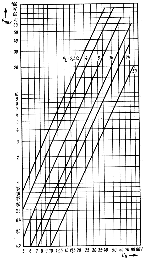
Bild 5. Zusammenhang zwischen P_{max} , U_b und R_L nach Gleichung 1
