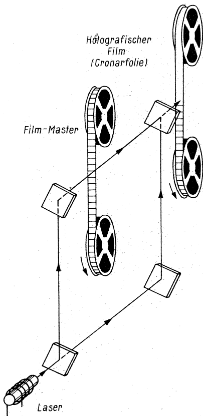
Bild 4. Herstellung des Hologramm-Masters aus dem Film-Master
