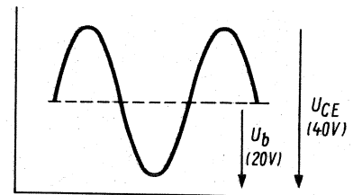
Rechts: Bild 3. Verhältnis von Speisespannung zur zulässigen Kollektoremitter-Spannung in einer Gegentakt-Endstufe
