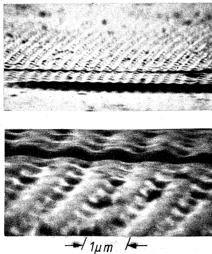
Bild 5. Elektronenmikroskopische Aufnahme der Oberflächenstruktur einer holografischen Selectavision-Aufzeichnung
