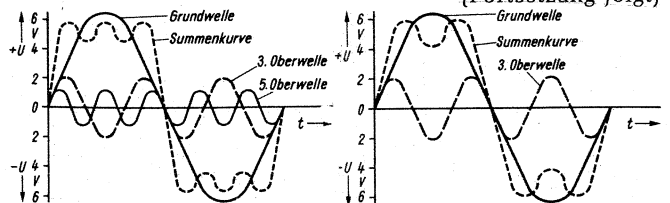
Bild 2.9. Aufbau von Rechteckwechselspannungen aus Oberwellen
