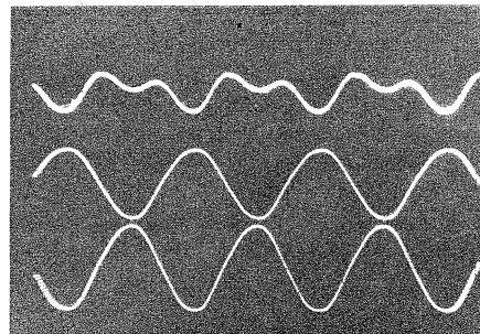
Bild 9. Bei Addition zweier Sinusspannungen mit einem Phasenunterschied von \varphi = 180^\circ bleibt als Summe der Oberwellenanteil übrig. Um hier die Oberwellen besser sichtbar werden zu lassen, wurde dieser Eingang des Oszillografen wesentlich empfindlicher gemacht
