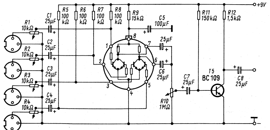
Bild 10. Vierkanalmischer für Phonoanwendung
