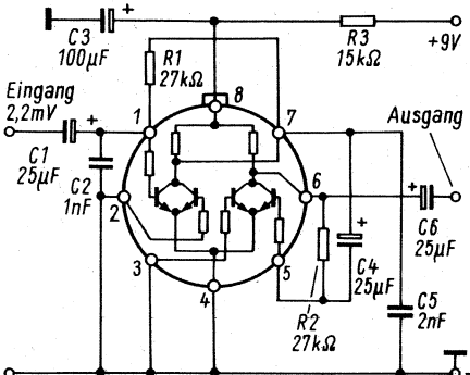
Bild 3b. Zweistufiger Wechselspannungsverstärker
