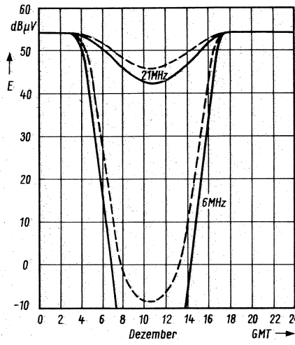
Bild 6. Berechnete Feldstärkekurven der Deutschen Welle für die Verbindung Jülich - Kigali (ausgezogen R = 100 , gestrichelt R = 5 )
