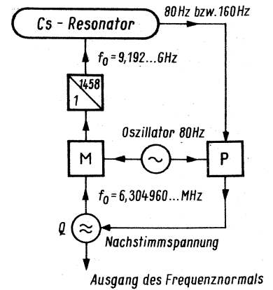
Rechts: Bild 4. Vereinfachtes Blockschaltbild eines absoluten Frequenznormals
