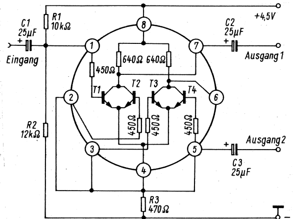
Bild 4a. Einstufiger Phasenaufspalter
