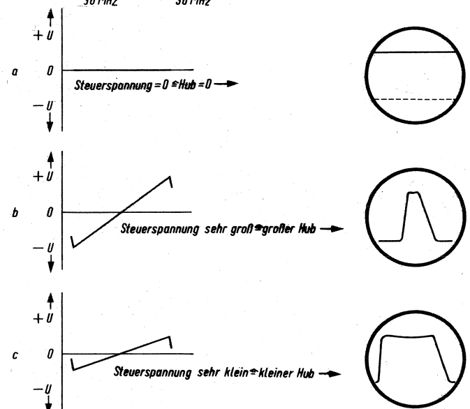
Bild 52a. Wobbelsteuerspannung = Null Bild 52b. Wobbelsteuerspannung zu groß Bild 52c. Wobbelsteuerspannung zu klein
