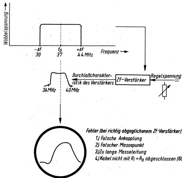
Bild 55. Falsche Durchlaufkurve durch Fehlanpassung des Wobblers
