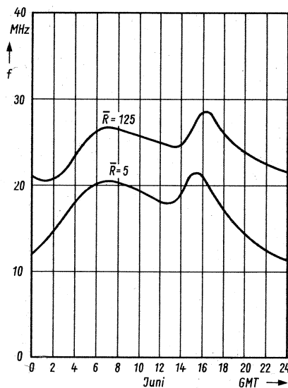
Oben: Bild 4. Funkprognose der Deutschen Welle für die Strecke Jülich - Indien für Juni und Dezember
