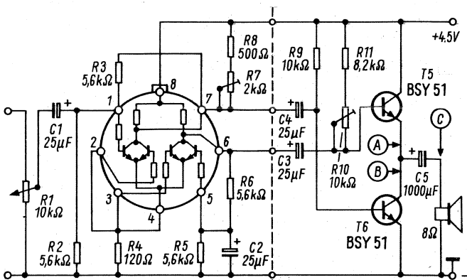
Bild 5a. Eisenloser Gegentakt-Endverstärker mit npn-Transistoren
