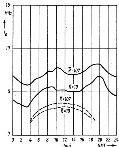
Bild 3. Gemessene senkrechte Grenzfrequenzen der E-Schicht (gestrichelt) und F-Schicht (ausgezogen) bei niedrigen und hohen Sonnenflecken im Juni und November
