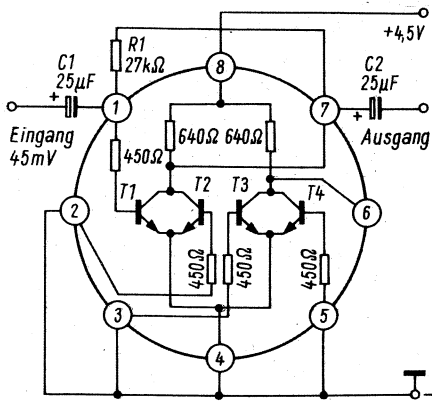
Bild 3a. Einstufiger Wechselspannungsverstärker
