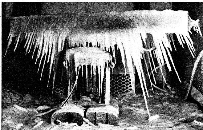
Bild 1. Vereiste Radarantenne in der Kältekammer, in der arktische Klimabedingungen simuliert und verschiedene Methoden zum Enteisen erprobt wurden
