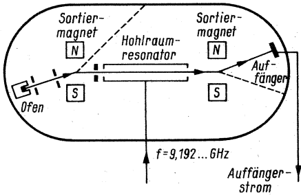
Bild 2. Prinzip des CS-Resonators
