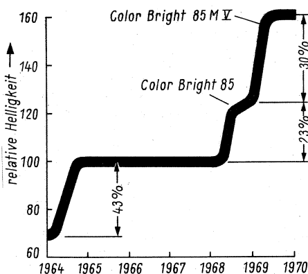
Zunahme der Bildhelligkeit der Sylvania-Farbbildröhren seit dem Jahr 1964
