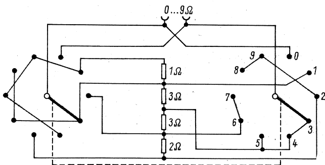
Schaltungsvorschlag für eine Widerstandsdekade mit vier Widerständen
