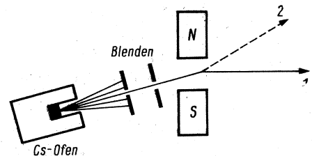
Bild 1. Aufspaltung eines Atomstrahls von Caesium-Atomen im inhomogenen Magnetfeld
