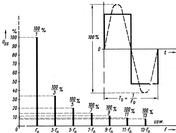
Bild 2.8. Frequenzen und Amplituden der Oberwellen einer Rechteckwechselspannung
