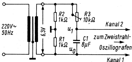
Bild 8a. Phasenschieber für Spannungen mit einer Frequenz von 50 Hz
