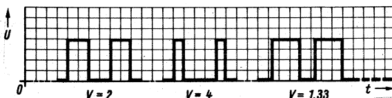
Bild 2.5. Rechteckpulse gleicher Periodendauer mit verschiedenem Tastverhältnis
