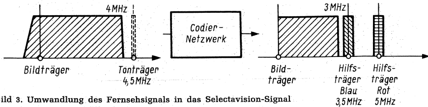
Bild 3. Umwandlung des Fernsehsignals in das Selectavision-Signal
