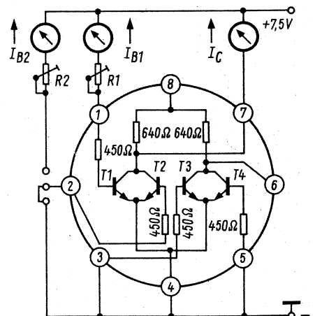
Bild 2. Prüfschaltung zum Aufnehmen der wichtigsten Kenndaten
