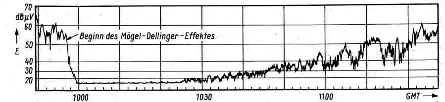
Bild 7. Feldstärkeregistrierung der Sendung der Deutschen Welle nach Japan auf 15 245 kHz. Aufgezeichnet von Oy. Yleisradio Ab. Helsinki am 5. 6. 1969
