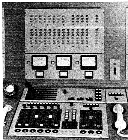
Teilaufnahme des Tisches für die internationale Regie (Intervision, Eurovision) mit Töneinstellern, Aussteuerungskontrolle und Vierdraht-Vermittlung für Fernsprechen (Aufn.: W. Franz KG, Lahr)
