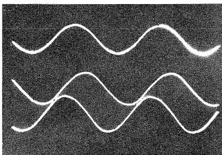
Bild 8c. Vektorielle Addition zweier gegeneinander phasenverschobener Sinusspannungen; unten = u_0 , Mitte = u_1 , oben = u_0 + u_1
