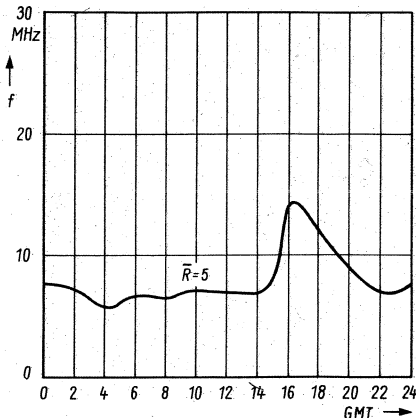
Bild 9a. Funkprognose der Deutschen Welle für die Linie Jülich - Nordamerika (West) Monat Januar
