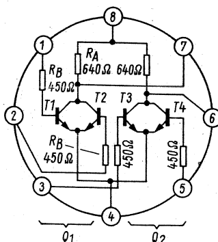
Bild 1b. Innenaufbau der integrierten Schaltung (Realschaltung)
