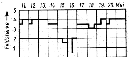
Bild 8. Feldstärke der Frequenz 6100 kHz, gemessen von der Empfangsstation der CBC in Ottawa
