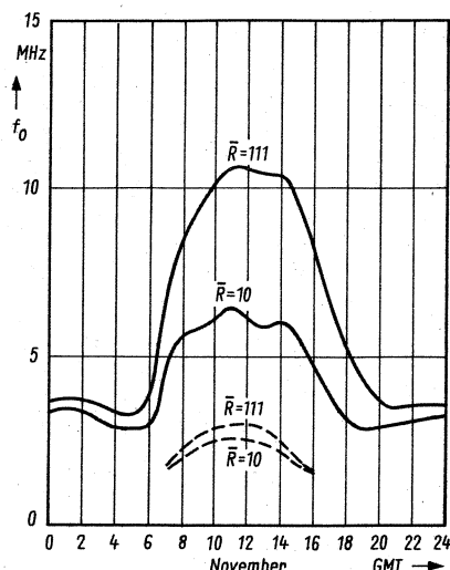
Bild 3. Gemessene senkrechte Grenzfrequenzen der E-Schicht (gestrichelt) und F-Schicht (ausgezogen) bei niedrigen und hohen Sonnenflecken im Juni und November
