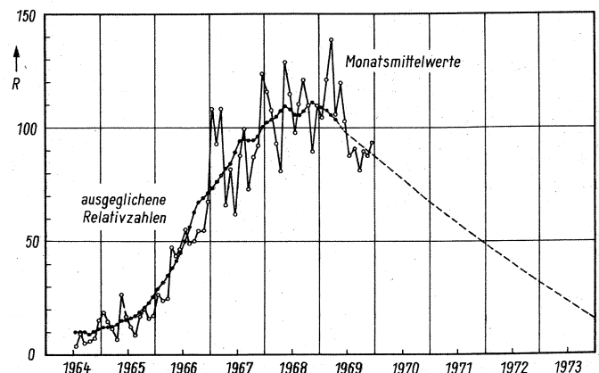
Bild 2. Sonnenfleckenzyklus Nr. 20
