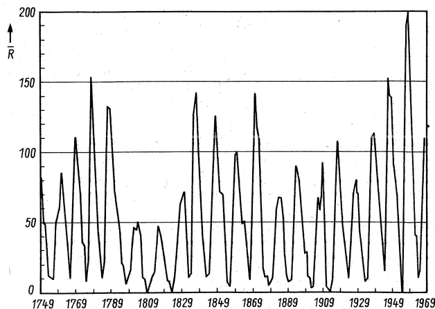
Bild 1. Sonnenfleckenzyklen von 1749 bis 1969
