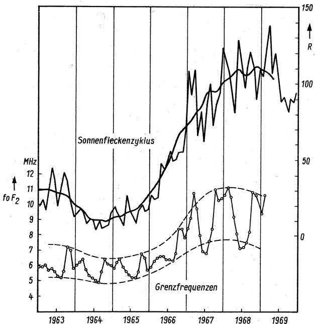
Bild 5. Vergleich der gemessenen Grenzfrequenzen der F-Schicht mit dem Sonnenfleckenzyklus
