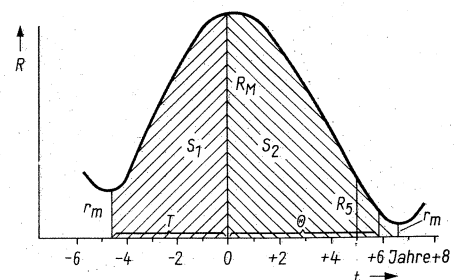
Bild 10. Schematische Darstellung eines Sonnenfleckenzyklus
