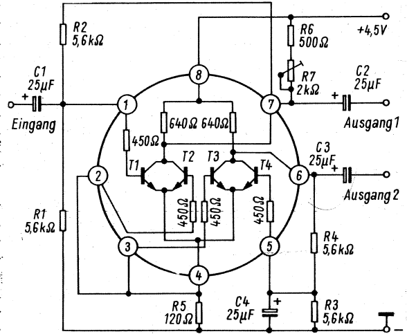
Bild 4b. Zweistufiger Phasenaufspalter
