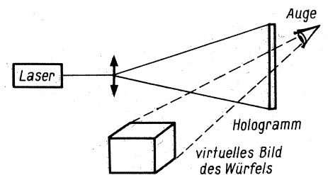
Bild 2. Rückgewinnung des dreidimensionalen virtuellen Bildes aus dem mit kohärentem Licht durchleuchteten Hologramm
