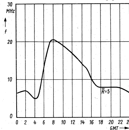
Bild 9b. Funkprognose der Deutschen Welle für die Linie Jülich - Neuseeland Monat Januar
