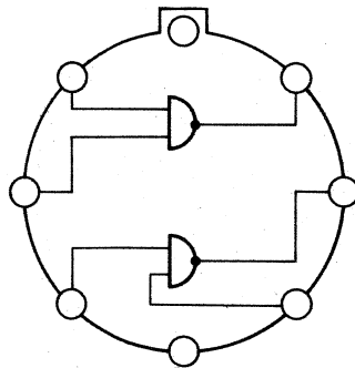
Bild 1a. Der Baustein RTL 914 von SGS mit der in der logischen Schaltungstechnik üblichen Darstellungstyp
