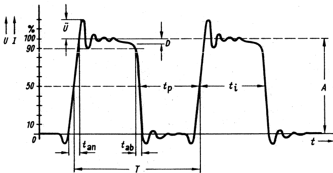
Bild 2.7. Kenngrößen der nichtidealen Rechteckimpulsfolge
