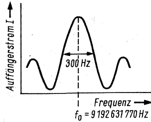
Bild 3. Resonanzkurve des CS-Resonators
