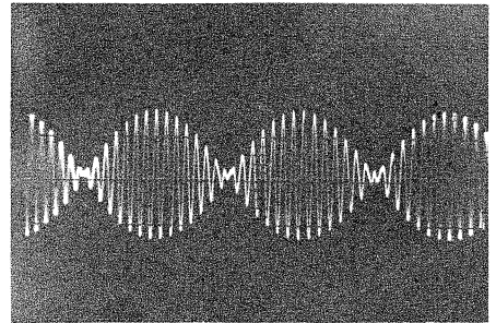
Bild 7b. Schwebung durch Mischung von f_1 und f_2
