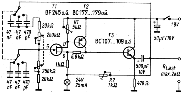
Schaltung des handlichen Sinusgenerators
