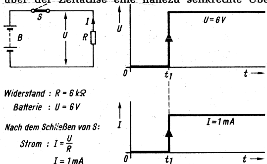
Bild 2.1. Spannungssprung und Stromsprung
