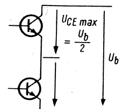
Rechts: Bild 4. Verhältnis von Speisespannung zur zulässigen Kollektoremitter-Spannung in einer übertragerlosen Endstufe
