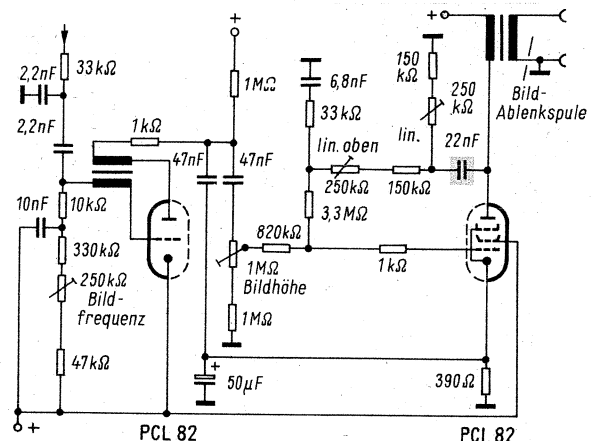
Durch einen Schluß des 22-nF-Kondensators wurde nur ein Teil des Bildablenksignales auf das Steuergitter der Röhre PCL 82 rückgekoppelt
