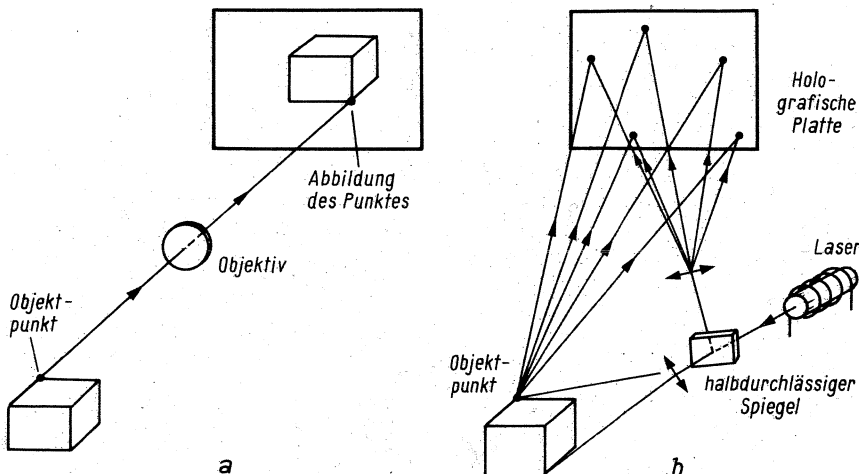
Bild 1. Während der Objektpunkt bei der fotografischen Aufnahme (a) nur eine Stelle der lichtempfindlichen Filmschicht schwärzt, ist im Hologramm (b) der Objektpunkt in jeder Stelle des Interferenzbildes enthalten
